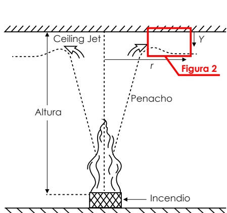
Figura 1: Interacción Penacho-Techo.
