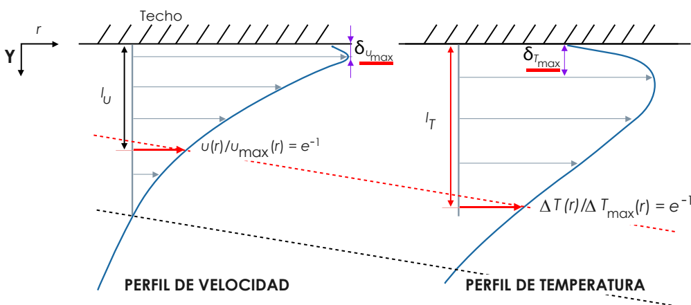
Figura 2: Perfil de Velocidad y Temperatura en el Ceiling Jet iii
